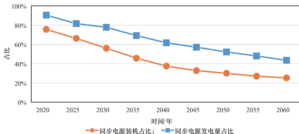
图1 同步电源装机及发电量占比的变化趋势
